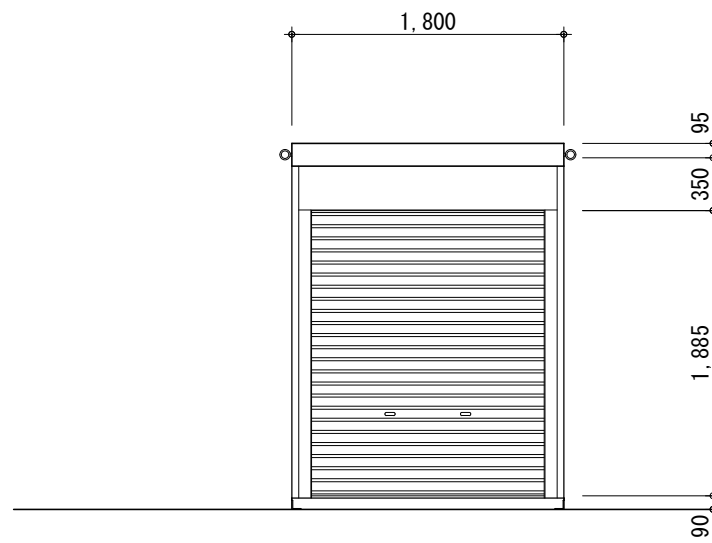
立面図 1:50
