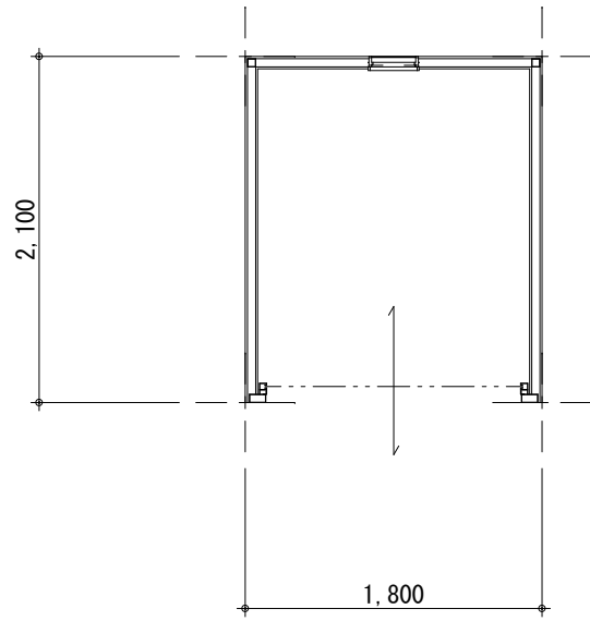
平面図 1:50
