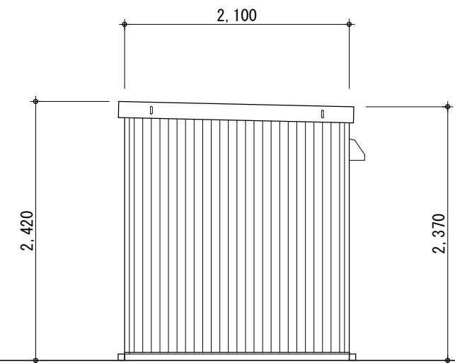
立面図 1:50
